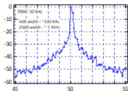
输出光谱
