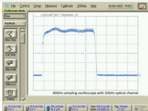
脉冲形状@2000mA
