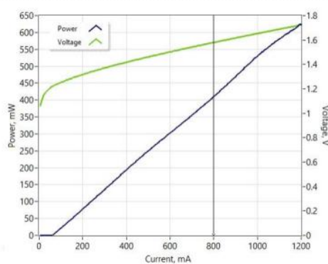
光电流电压特性
