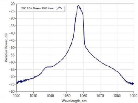
光谱 (分辨率 200pm)
