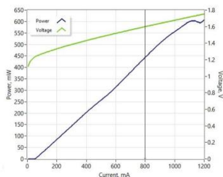
光电流电压特性
