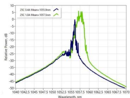
光谱(res. 200pm)
