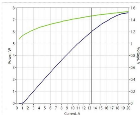
光-电流-电压特性
