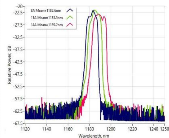
光谱 (分辨率 1nm)
