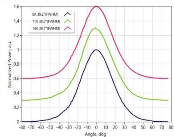
快轴远场
