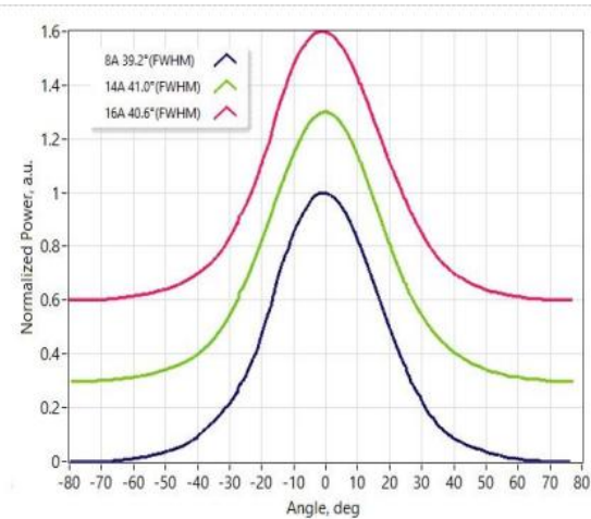
快轴远场
