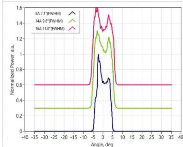
慢轴远场
