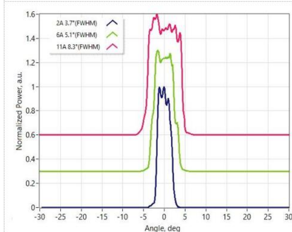
慢轴远场
