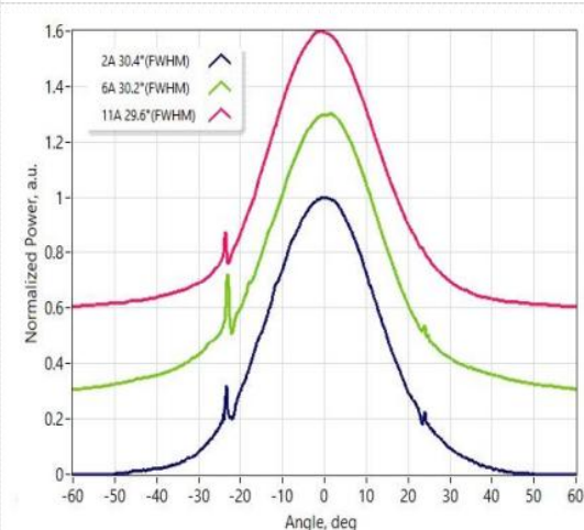
快轴远场
