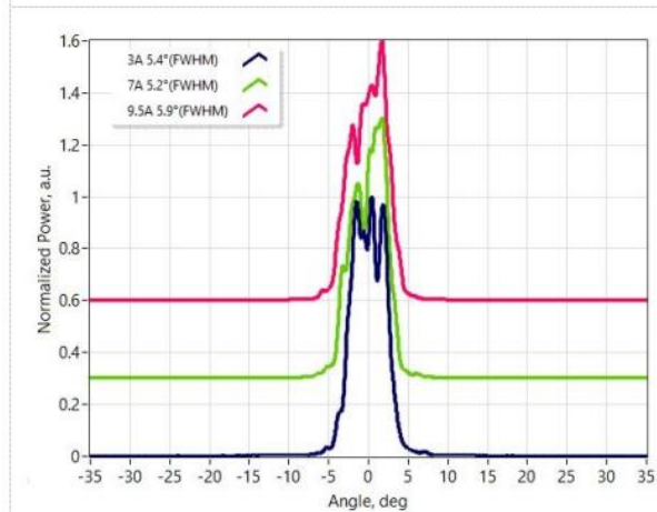
慢轴远场
