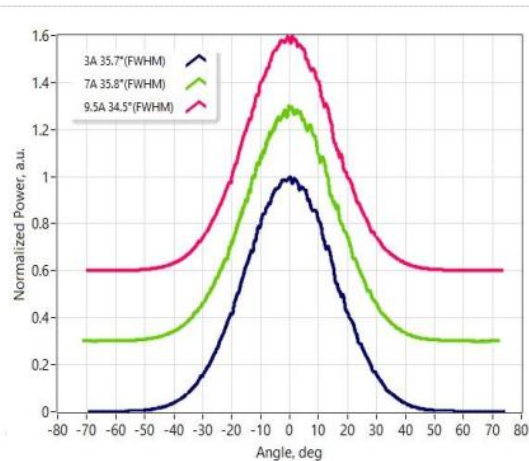
快轴远场
