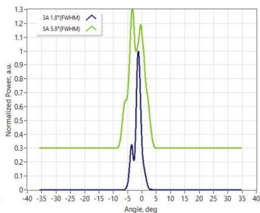
慢轴远场
