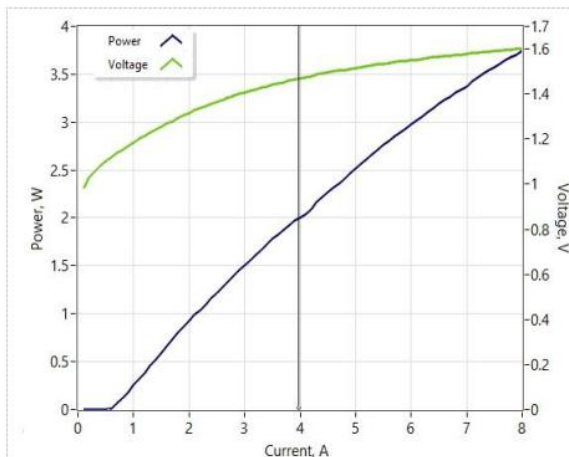
光-电流-电压特性
