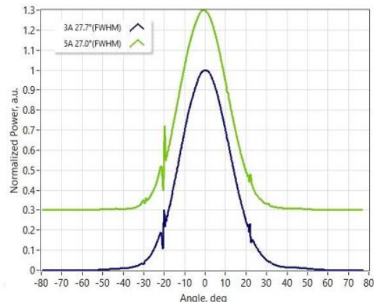
快轴远场
