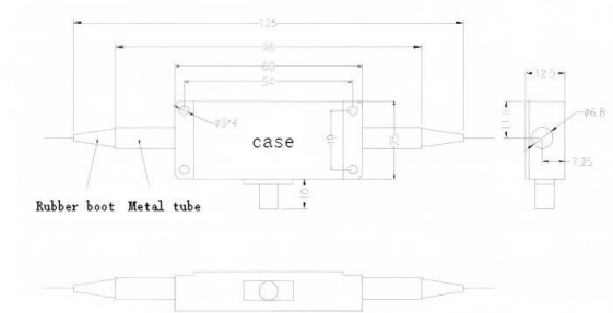
A:AOM Dimensions
