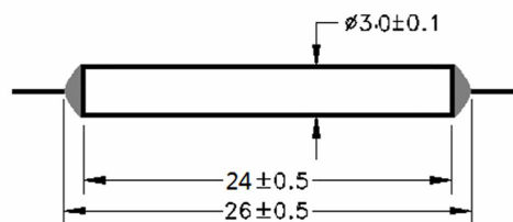
Mini fiber isolators
